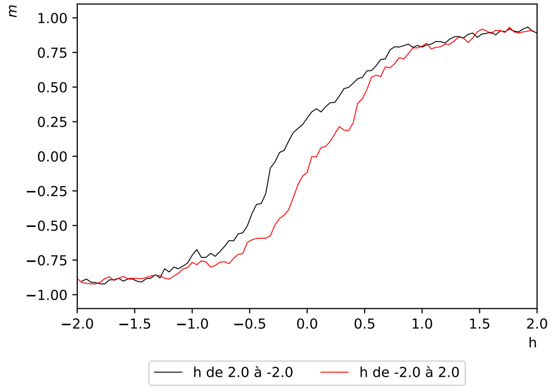
Hystérésis de l'aimantation - réseau de taille L=32 - champ magnétique d'amplitude h=2 à T=3.5
